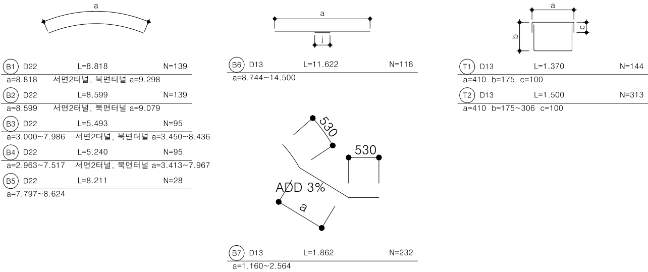
철근 집계표
